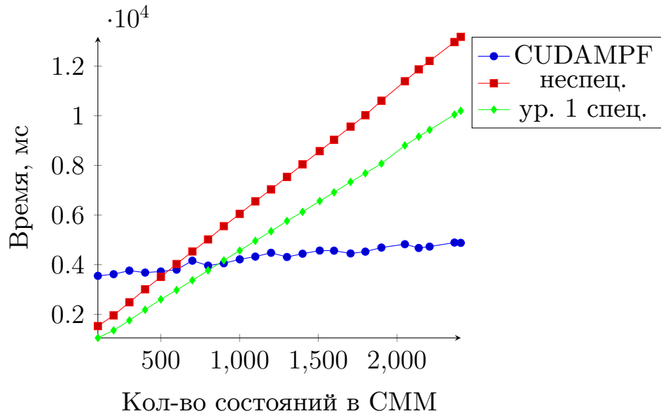
Рис. 7: GraphBLAS, 50 x 3500 наблюдений, меньше — лучше
