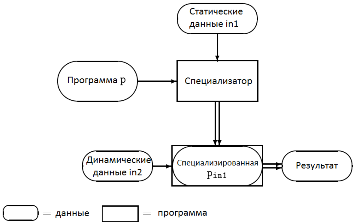
Рис. 2: Концептуальная схема специализации 1
