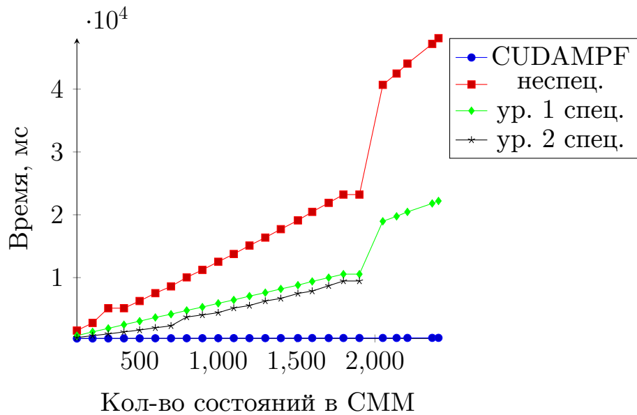
Рис. 11: cuASR, набор данных из БД PFAM, меньше — лучше
