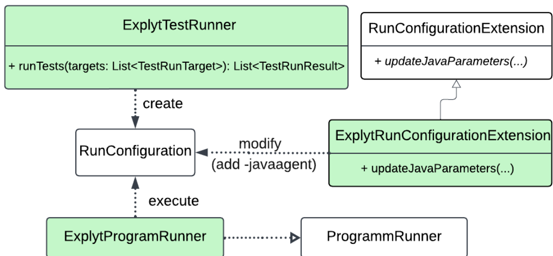
Рис. 2: Архитектура модуля test runner
