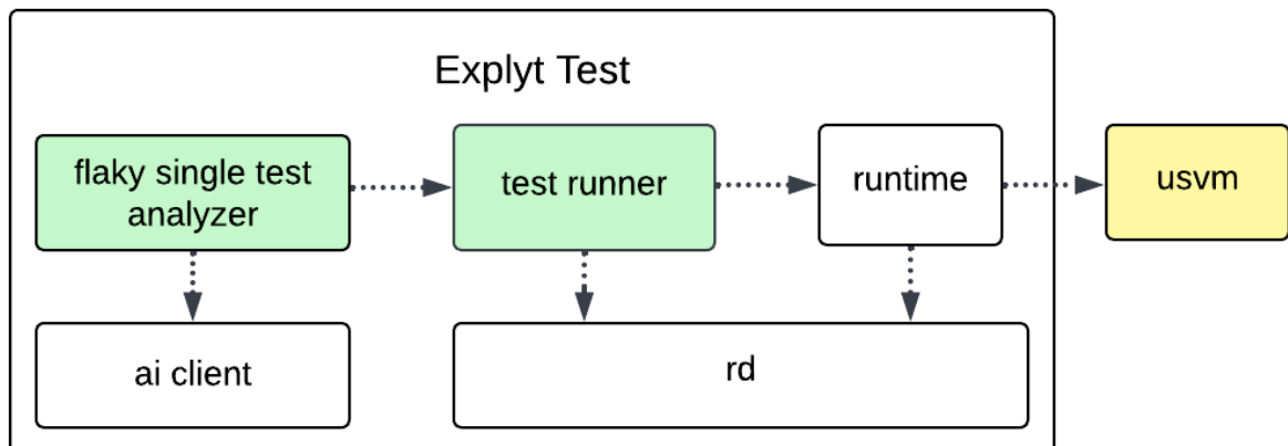
Рис. 1: Зависимость модулей в Explyt Test. Зеленым отмечены те, что были реализованы в данной работе. Желтым — те, в которые были внесены изменения
