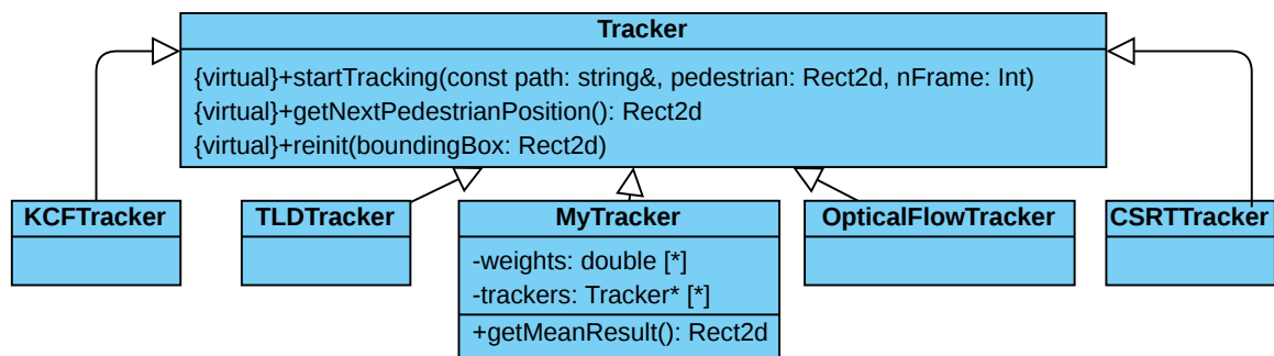
Рис. 2: UML-диаграмма классов текущей версии трекера
